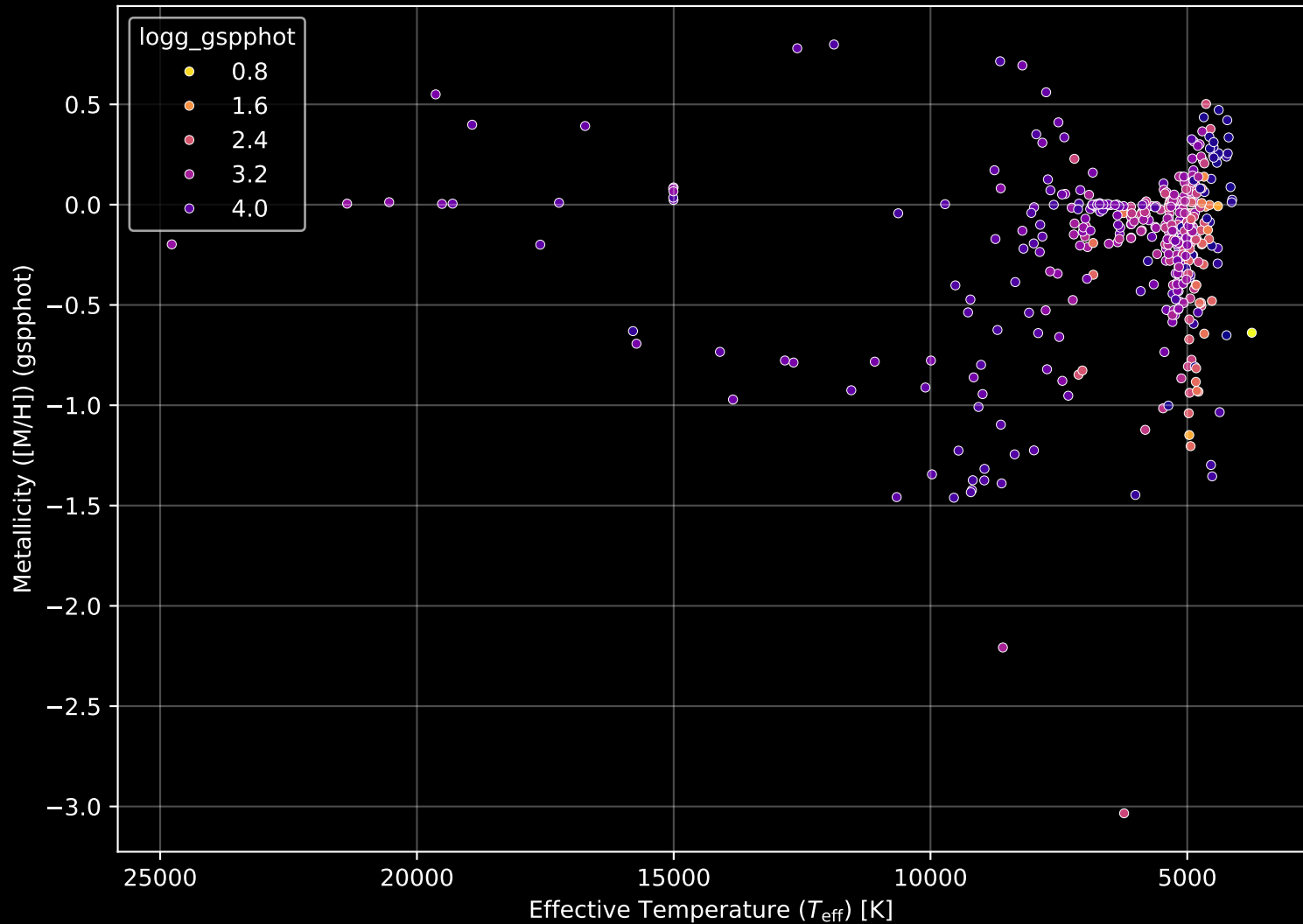
APOGEE DR17 Field: [HD46375] Stellar Population Parameters (n= 425)
